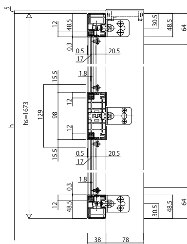
A-A断面
