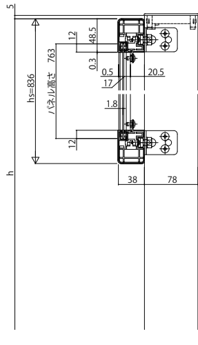
A-A断面
