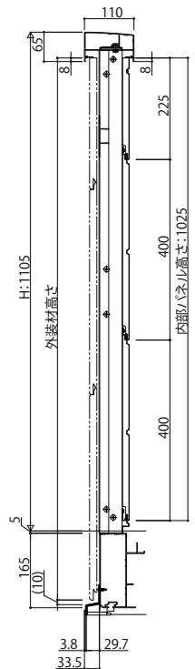
「外壁同仕上げ」(胴差し納まりのみ)
