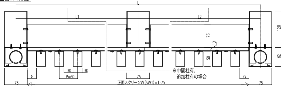
■正面スクリーン H寸法範囲
