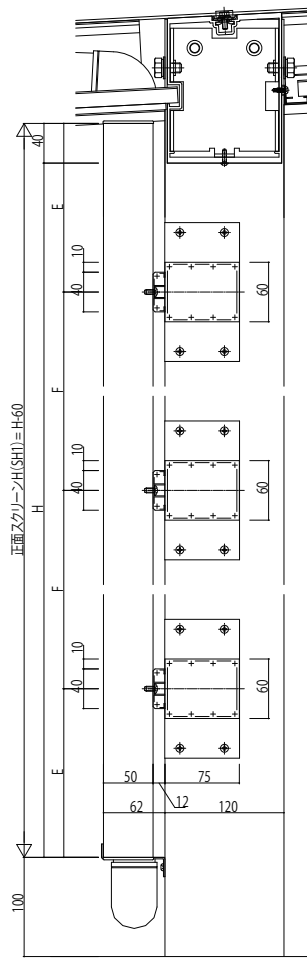
A-A断面
