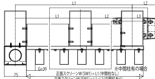
全面(C-C断面)
