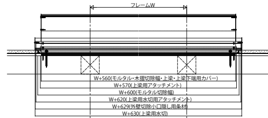
B-B断面図(柱部)
