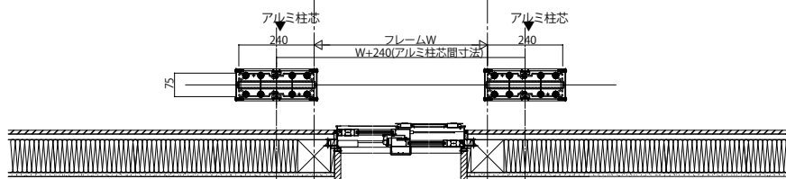
C-C断面図(下梁部)
