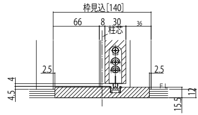
140mm見込
