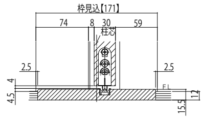
171mm見込
