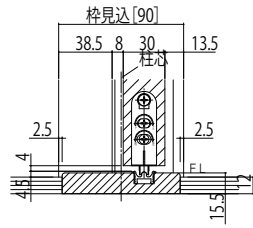
90mm見込
