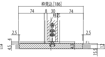
186mm見込
