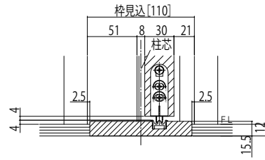
110mm見込
