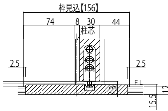
156mm見込
