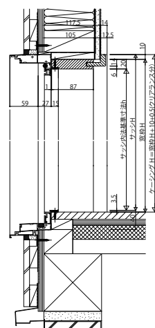
ケーシングタイプ フラットケーシング 通風ドア
