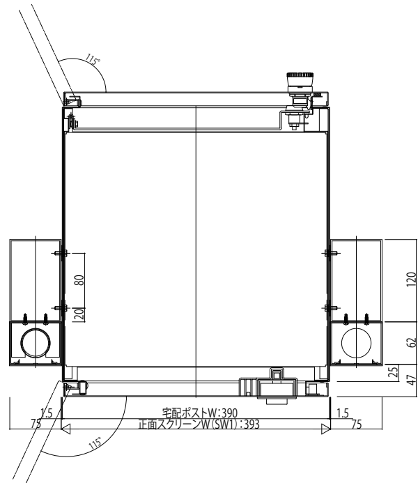
●D-D断面(追加柱)
