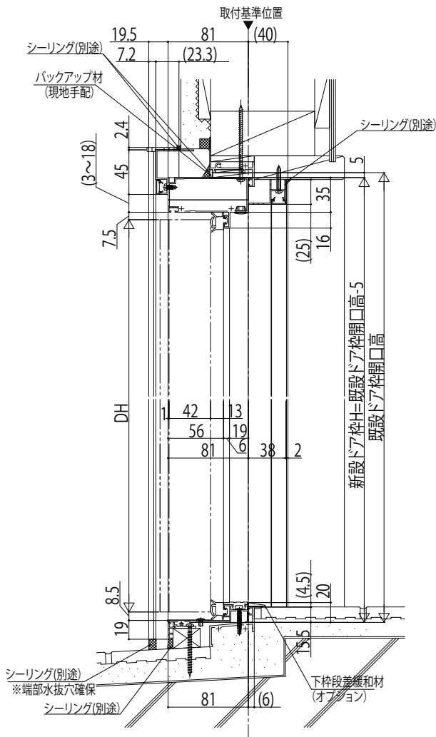
●ドア部 D4仕様(A-A´ 断面)
