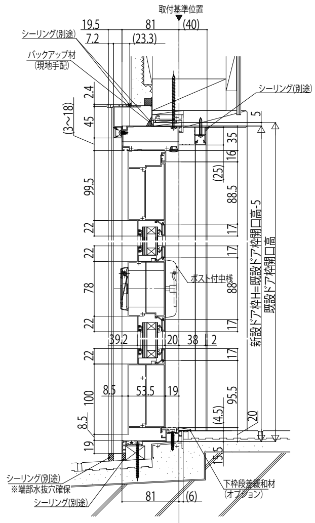
●袖部 D4仕様(B-B´ 断面)
