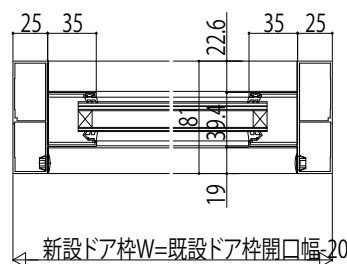
●両袖FIX枠 ランマ部 D4仕様 (K-K'断面)
