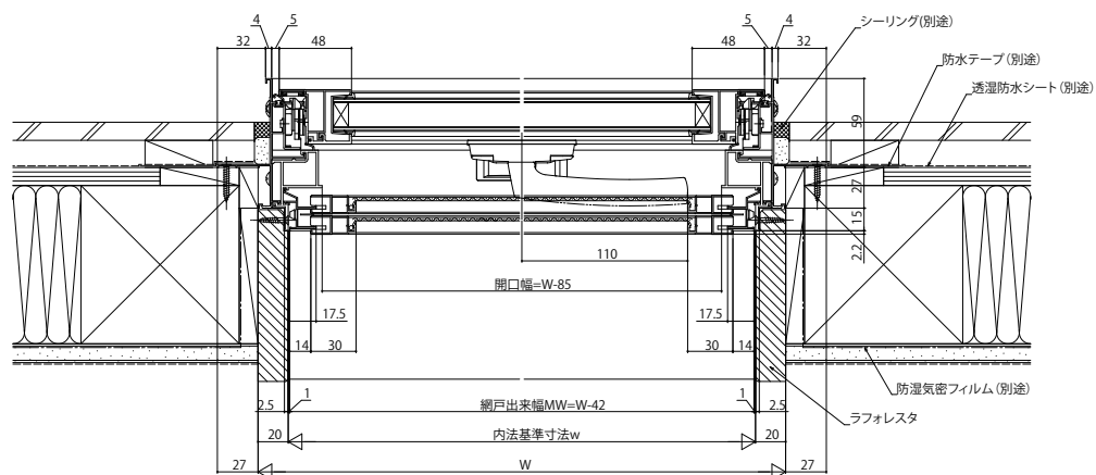
W ≤ 350の場合
