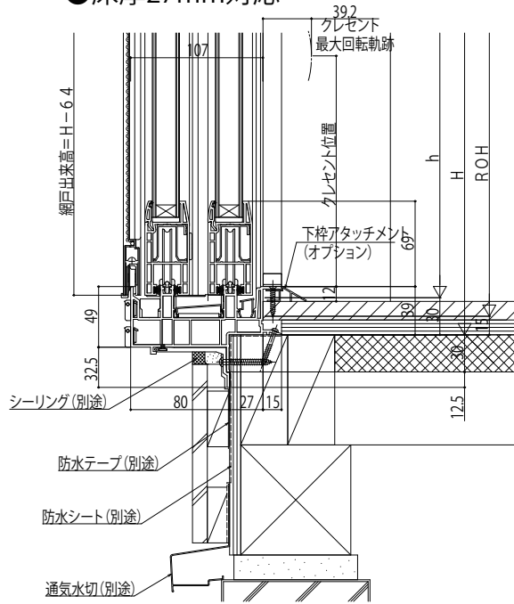
内障子開閉の場合 (外障子固定)
