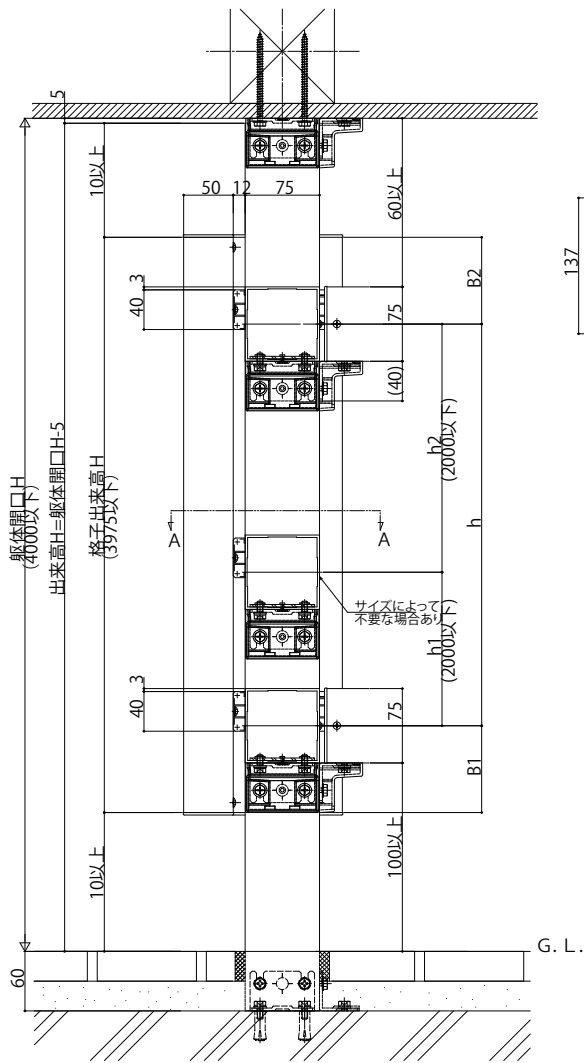
B-B断面
