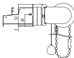
A-A断面図
