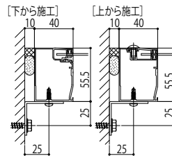
A-A断面
