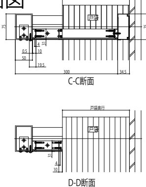
D-D断面
