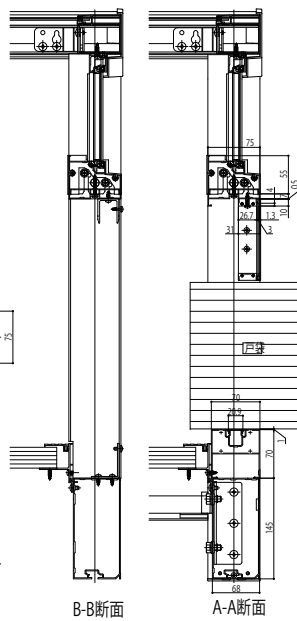
B-B断面
