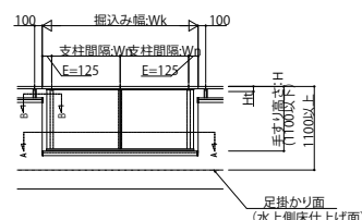
外観姿図
