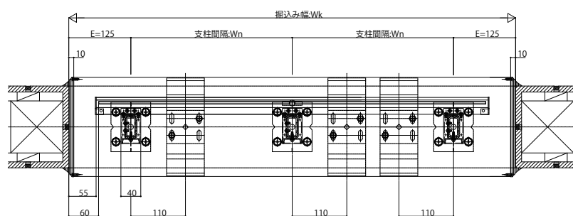
A-A断面
