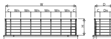
外観姿図
