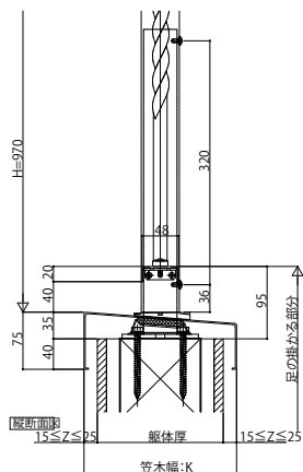
本図は笠木幅K=200(躯体厚=165)を示す。
