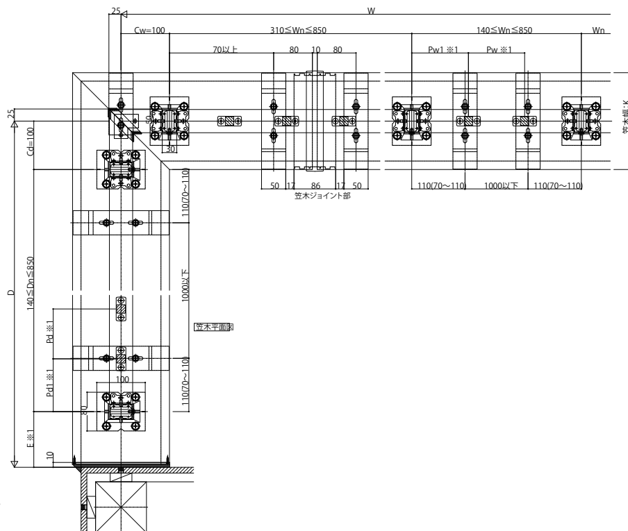
本図は笠木幅K=200(躯体厚=165)を示す。
