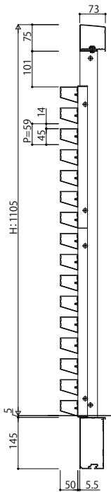
●台形格子
