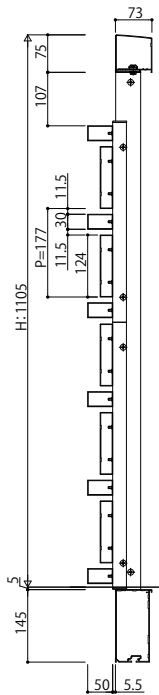
●組合せ格子
