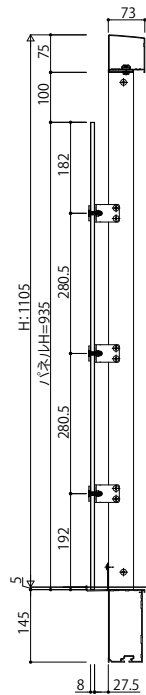
●DPG/パネル
