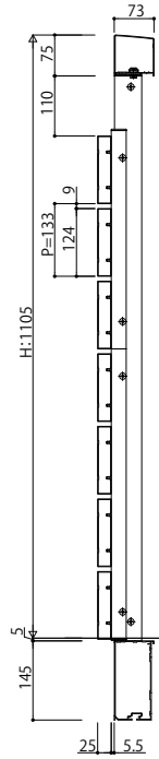
●横格子
