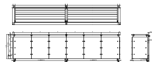
●DPGパネル【連結】
