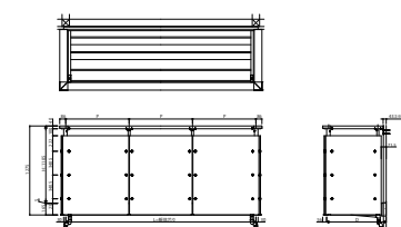
●DPGパネル【単体】
