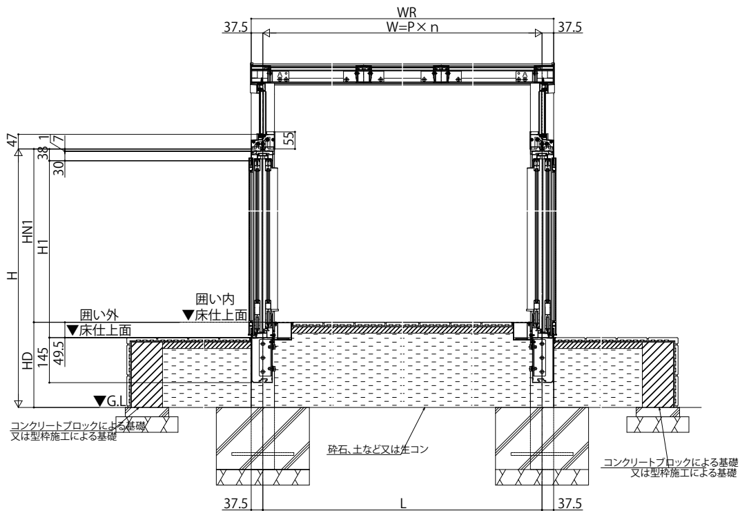
A-A断面
