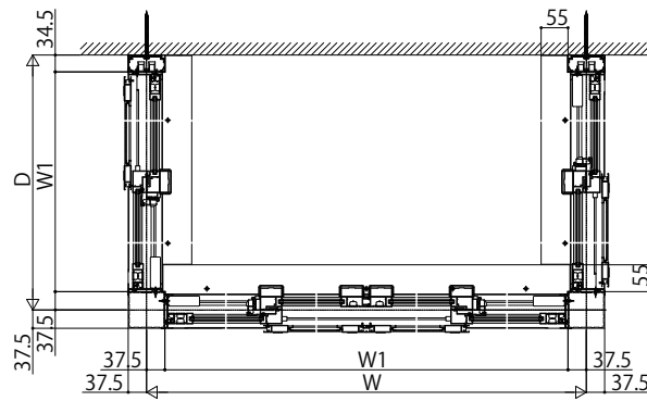
C-C断面
