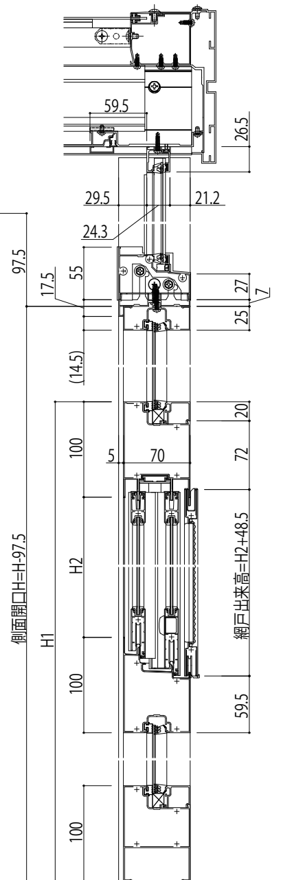
側面 高窓 (B-B断面)
