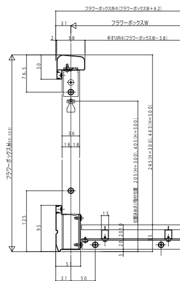
●正面図(A-A断面)
