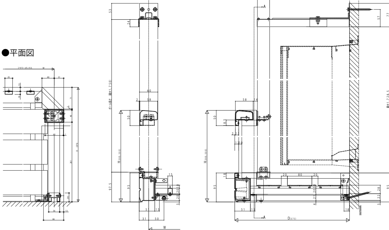
●正面図(A-A断面)
