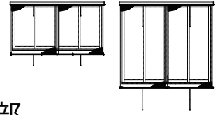
外観姿図
