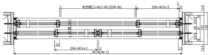
横格子デザイン 格子部寸法
