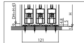
直付敷居の場合
