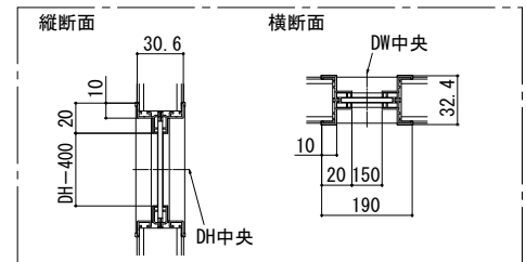
C11デザイン 採光部寸法
