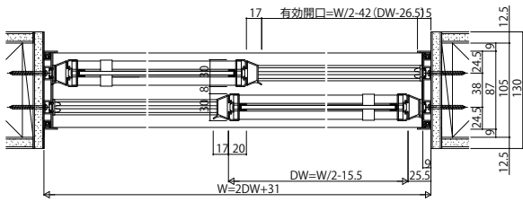
【E】引違い戸(2枚建)
