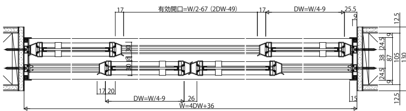
【G】引違い戸(4枚建)
