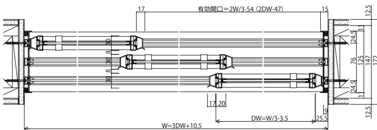
【F】引違い戸(3枚建)
