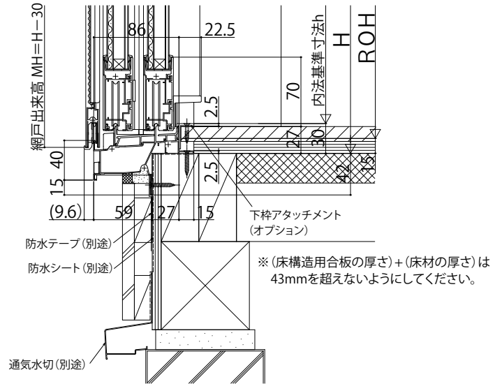
●単純段差下枠の場合
