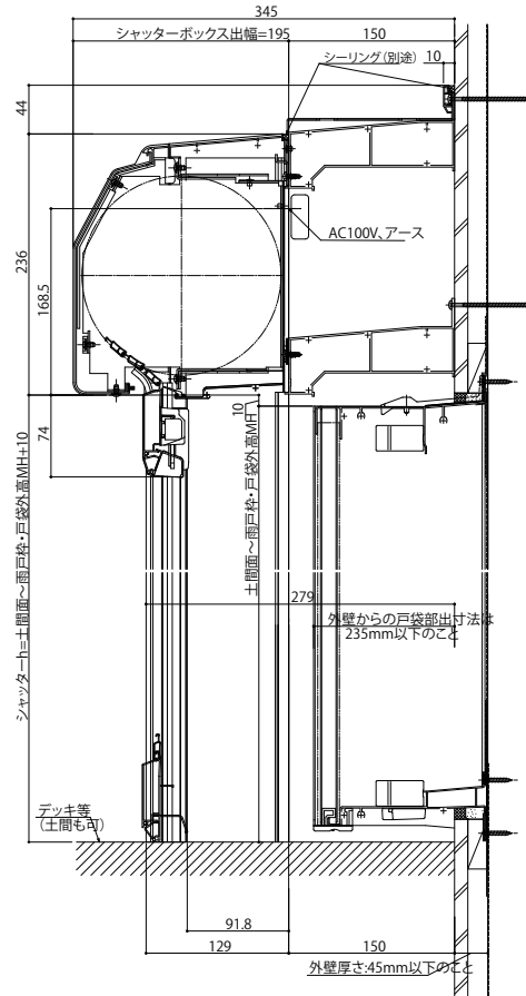
●戸袋側
