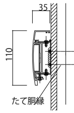
□R型 たて胴縁取付け
