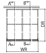
屋根平面図
