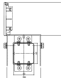
A-A断面図(1:1)
