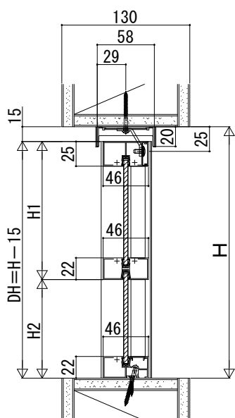
2段 FIX窓 (不均等)
