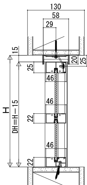
2段 FIX窓
