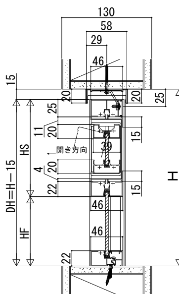
2段 すべり出し窓+FIX窓 (不均等)
