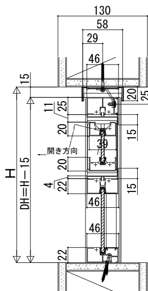
2段 すべり出し窓+FIX窓
