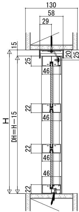
3段 FIX窓
