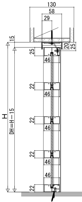
4段 FIX窓
