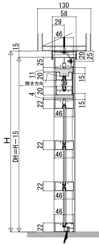
4段 FIX窓+すべり出し窓
