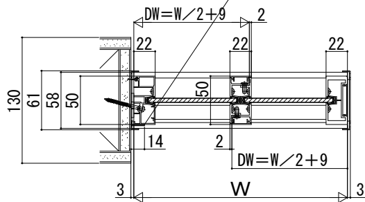
片側オープン納まり (左側壁) 2列 FIX窓部
