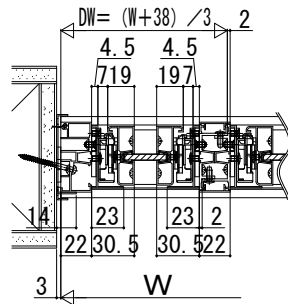
両側壁納まり 3列 すべり出し窓部
