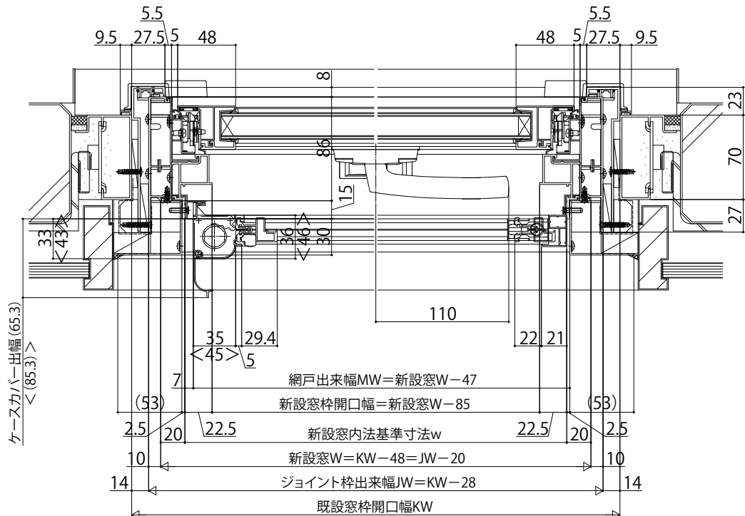
< >寸法は、新設窓W > 405の場合
