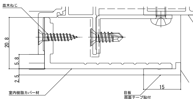
●たて枠納まり詳細図
