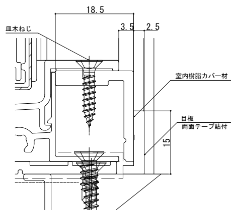
●下枠納まり詳細図
