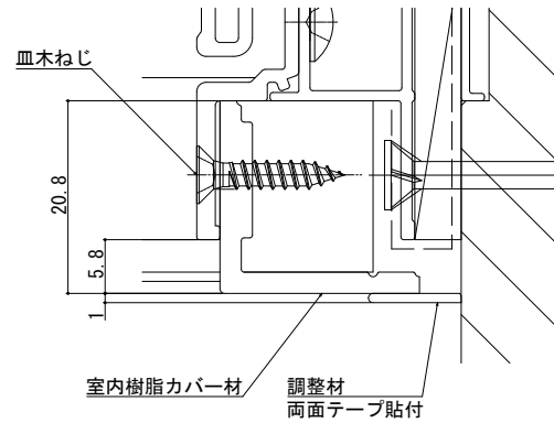
●たて枠納まり詳細図
