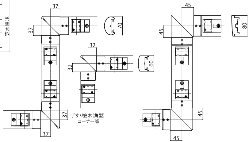
手すり笠木平面図
