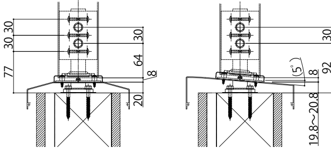
平笠木
