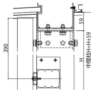
中間柱詳細 格子ユニット連結部
