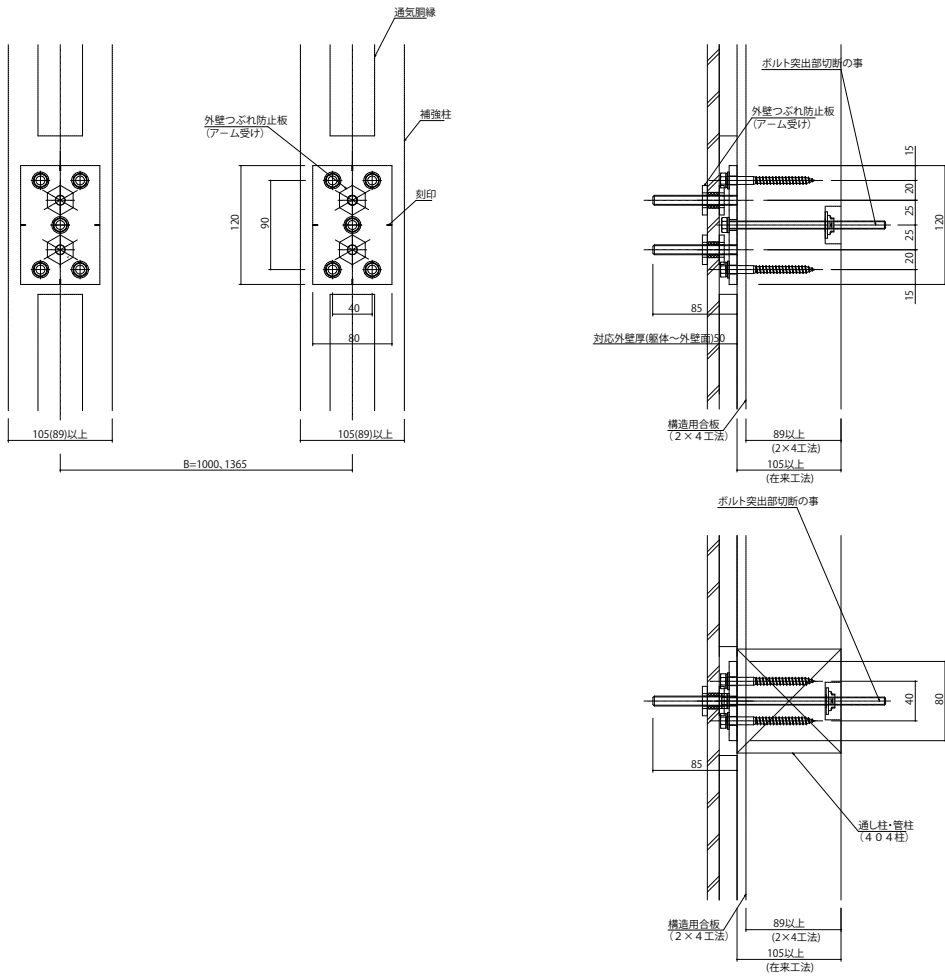
先付け金具
