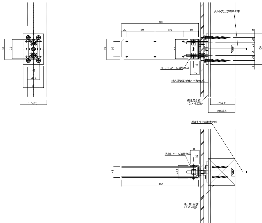
先付け金具+持ち出しアーム
