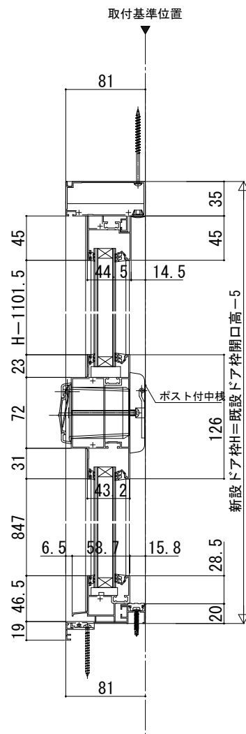
●袖部 D4仕様（B-B' 断面）
