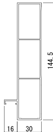
たて枠 (戸尻側)
