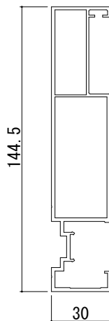
たて枠 (戸先側)
