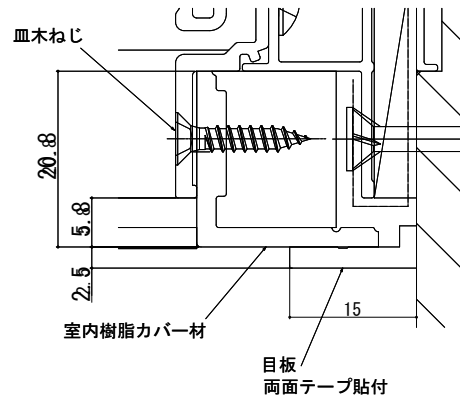
●たて枠納まり詳細図
