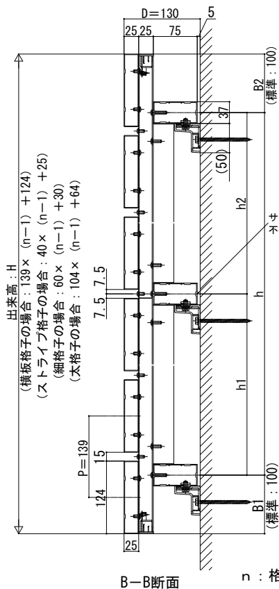
B-B断面
