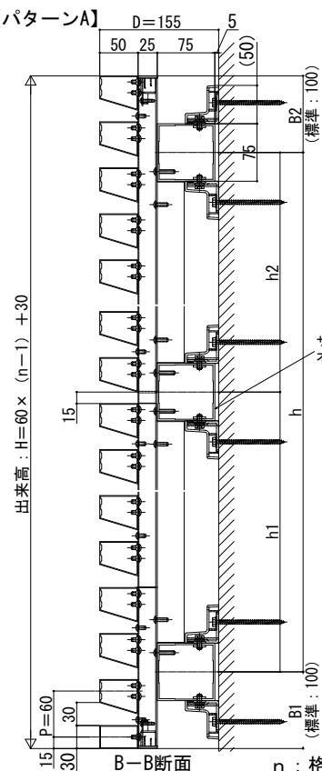
B-B断面
