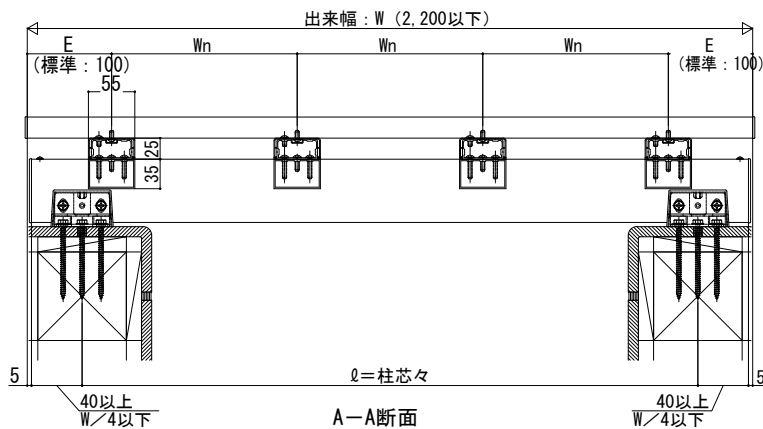
A-A断面
